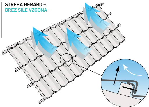
BETONSKA/ OPEČNA STREHA – SILA VZGONA
